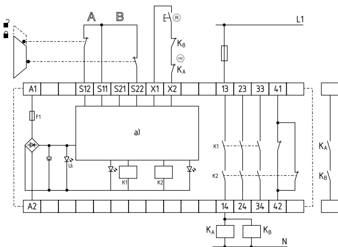
Fig. 2 a) Logica di controllo ® = Circuito di ripristino
