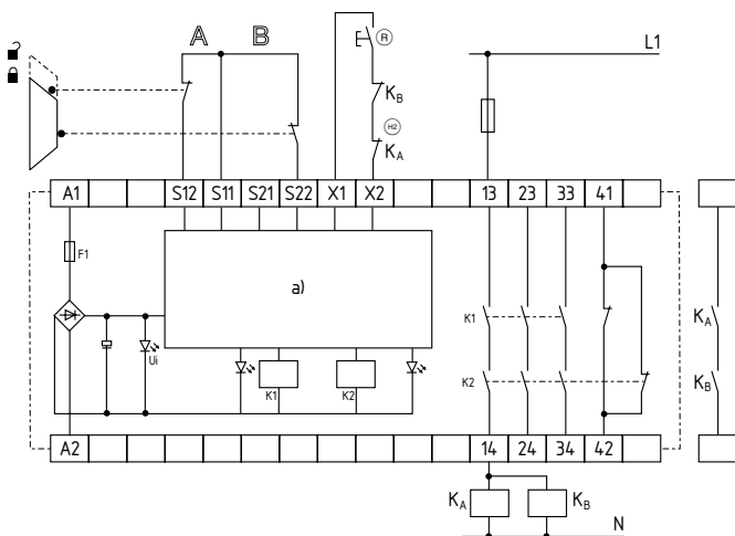
Afb. 2 a) Besturing ⊕ = Terugkoppeling
