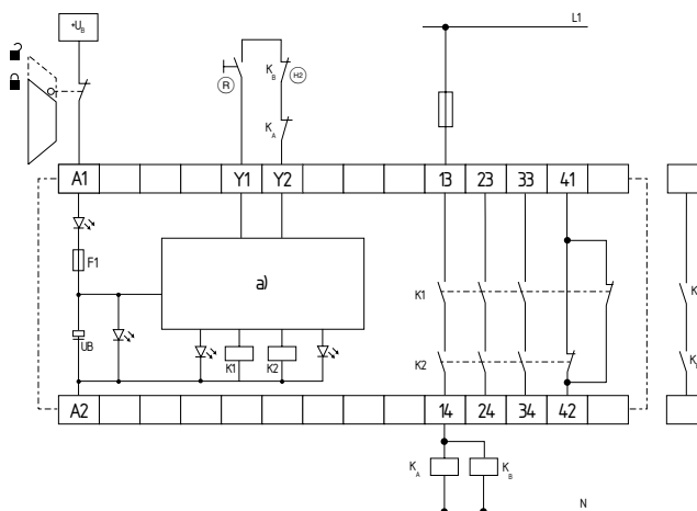
III. 2 a) Kontrollogik
