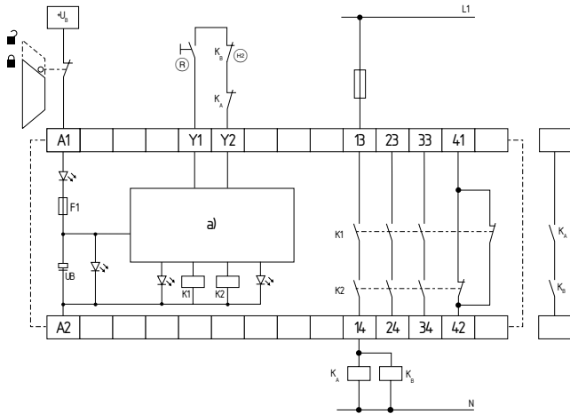
図2 a) 制御ロジック
