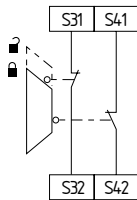
Fig. 12 SRB202CS, SRB202CS/T
