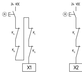
Fig. 5 côté gauche = niveau de déclenchement 1 côté droite = niveau de déclenchement 2 (SRB202CA, SRB202CS et SRB202CA/Q)
