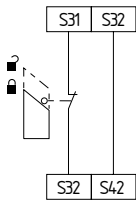
Fig. 11 SRB202CS, SRB202CS/T
