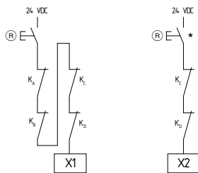
Fig. 6 côté gauche = niveau de déclenchement 1 côté droite = niveau de déclenchement 2 (SRB202CA/T, SRB202CS/T et SRB202CA/QT)
