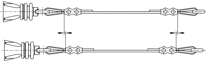
Figura 2: Deformação dos olhais
