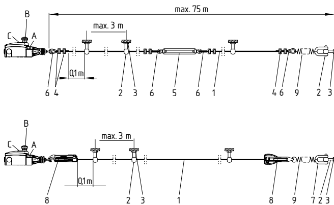
Rys. 2: Montaż komponentów
