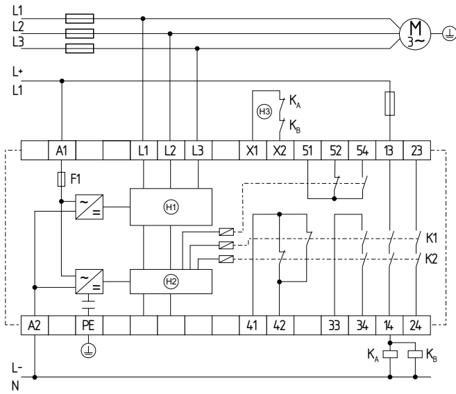
Fig. 4 (H1) = Procesamiento de señales (H2) = Monitorización (H3) = Circuito de realimentación
