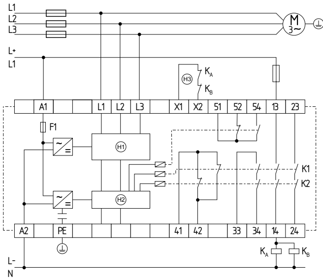
Fig. 4 (H1) = Tratamento do sinal (H2) = Monitorização (H3) = Circuito de retorno
