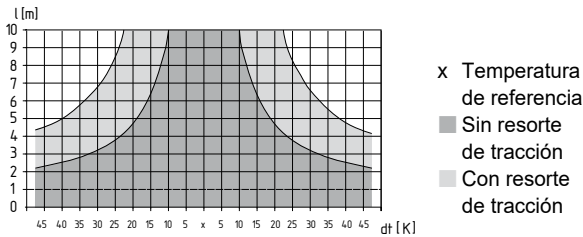
Figura 4: Longitud de cable máxima dependiendo de la temperatura, con o sin resorte de tracción.
