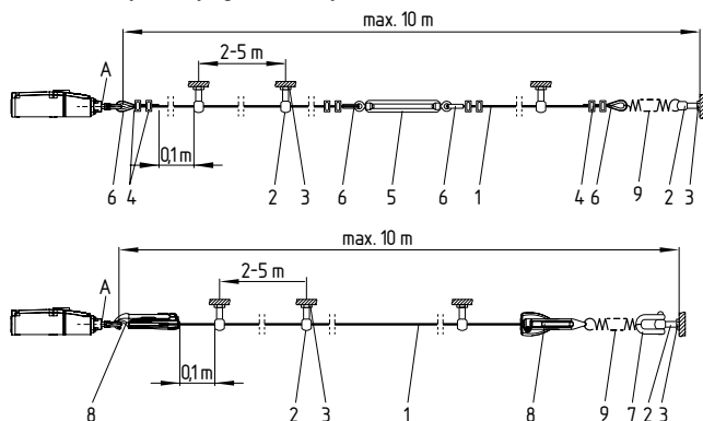
Rys. 2: Montaż komponentów
