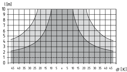
Rys. 4: Maksymalna długość linki w zależności od temperatury ze sprężyną kompensacyjną lub bez sprężyny
