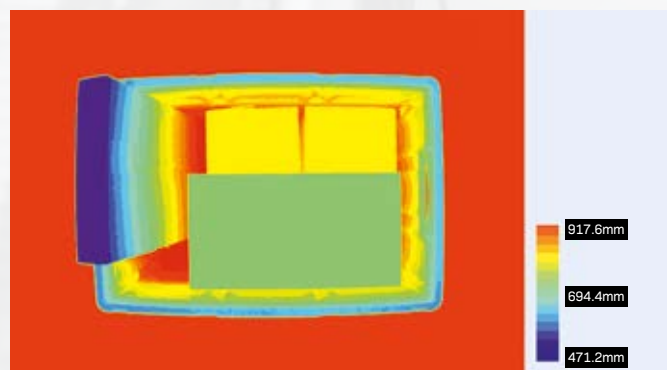
Dieptebeeld met 3D-camera AM-T100
