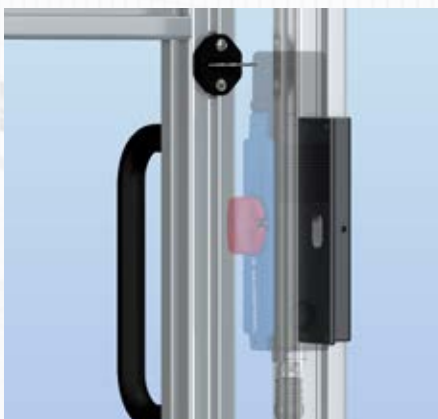
Haakse en rechte montageplaten voor aanbouw aan 40 mm profielen voor draai- en schuifdeuren
