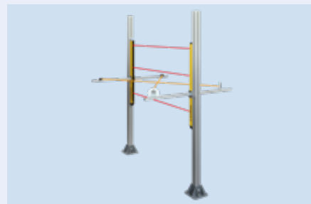
与方向无关的物料运输
