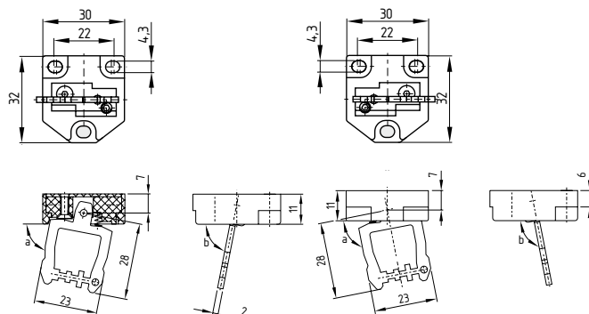
Beweeglijke bedieningssleutel B6L Beweeglijke bedieningssleutel B6R
