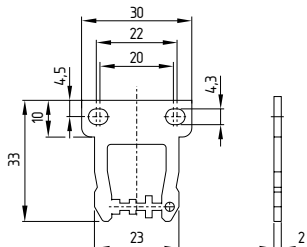
Rechte bedieningssleutel B1
