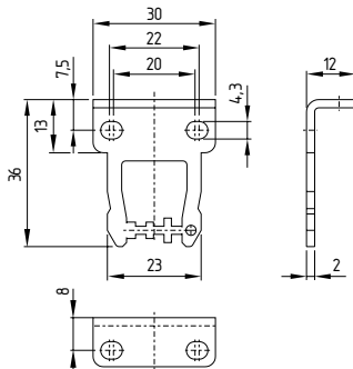
Haakse bedieningssleutel B5
